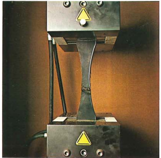
Kord bezi uygulanmış lastiğin instron cihazında kopma testi
